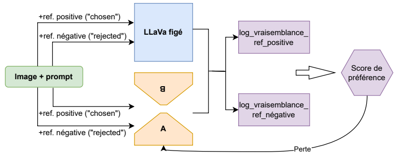
FIGURE 1 – Architecture proposée : Réglage des instructions de LLaVa avec LoRA et DPO
